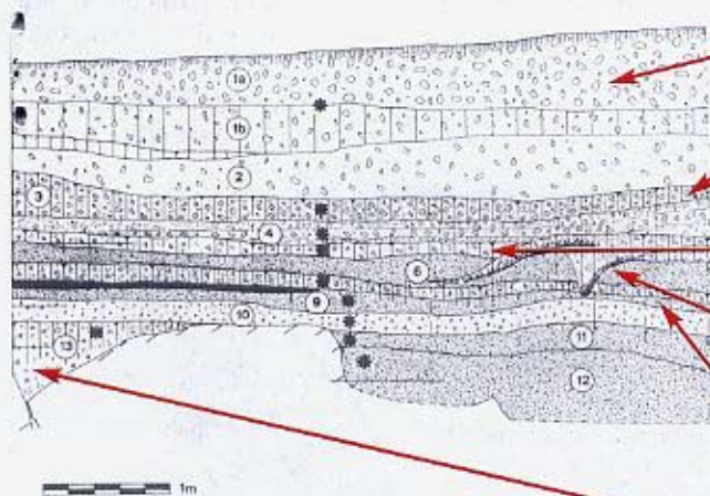
(Fig. 4) La stratigrafia della trincea a monte del masso in cui si aprono i ripari
